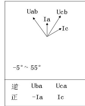
A、B相电压接反
