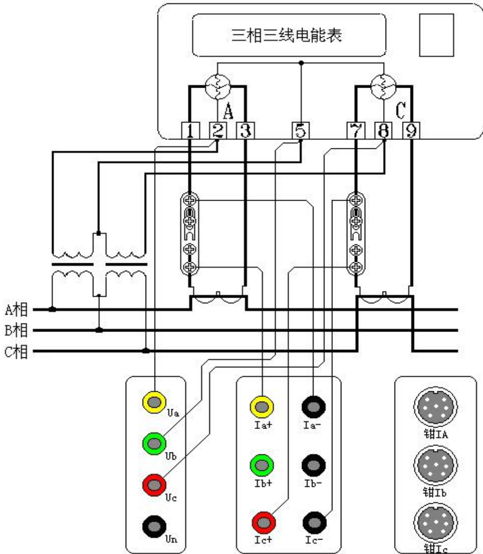
图二十四、三相三线高压计量表计直接接入测试
